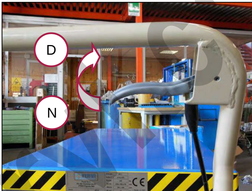
Figura 8 – Dettaglio leva di discesa del carrello.
