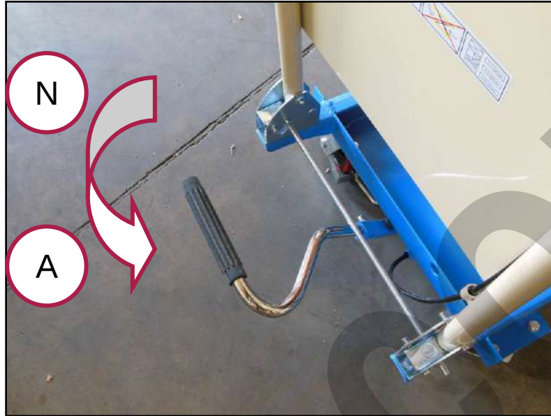
Figura 9 – Dettaglio pedale di sollevamento del carrello.
