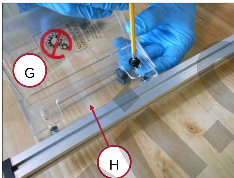
Figura 15 – Montaggio riparo
