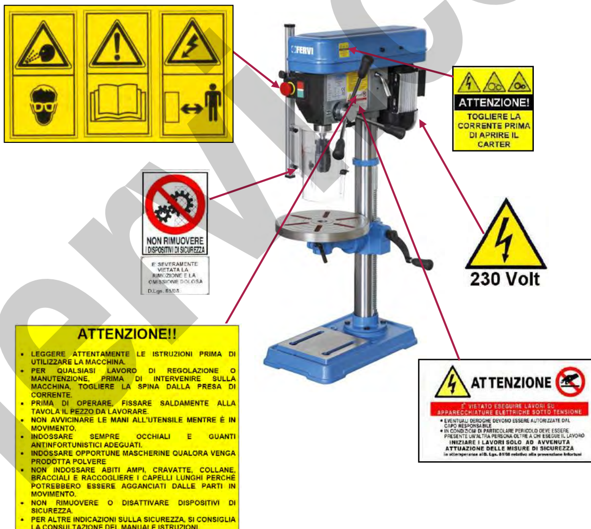
Figura 21 – Pittogrammi
