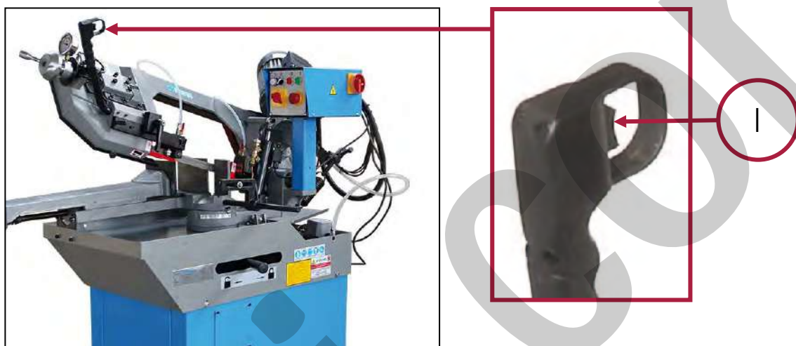
Figura 5 – Pulsante di avviamento lama, in modalità manuale.
