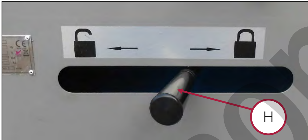
Figura 4 – Leva di bloccaggio della testa.
