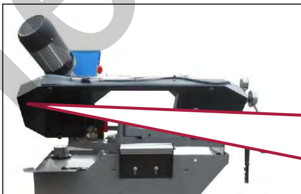
Figura 30 – Smontaggio del carter di protezione lama.
