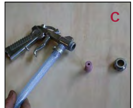
Figura 16 - Smontaggio dell'ugello della pistola sabbiatrice.
