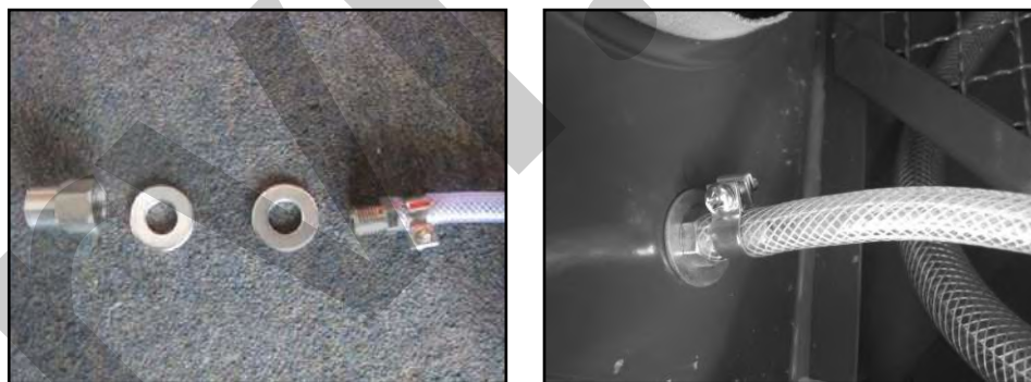
Figura 5 - Collegamento dell'aria compressa.
