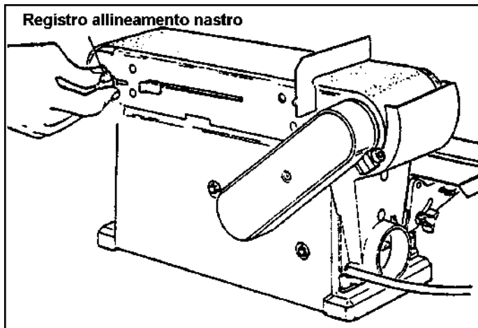
Figura 14 – Allineamento del nastro abrasivo.
