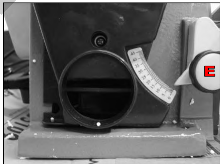
Figura 21 – Inclinazione della tavola di lavoro.
