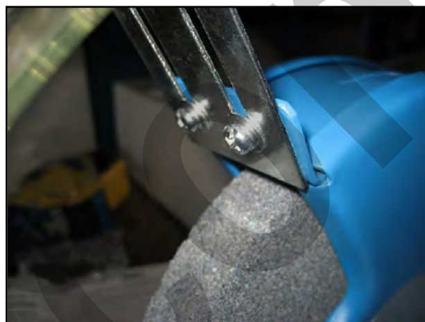
Figura 5 – Montaggio degli schermi di protezione.
