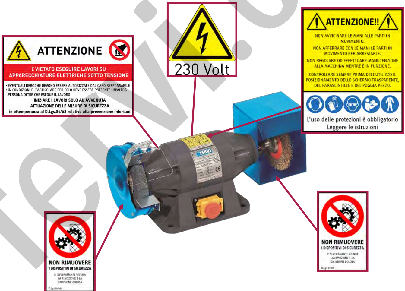
Figura 3 – Pittogrammi di segnalazione
