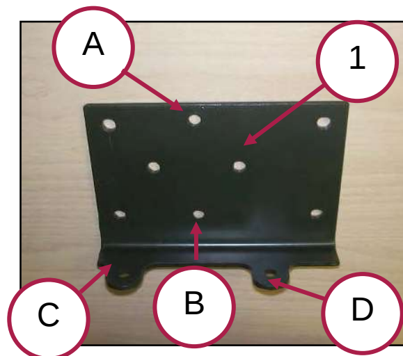
Figura 6 – Piastra di collegamento.
