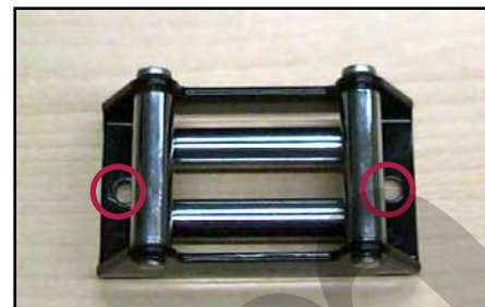
Figura 7 – Guida cavo / fine corsa.
