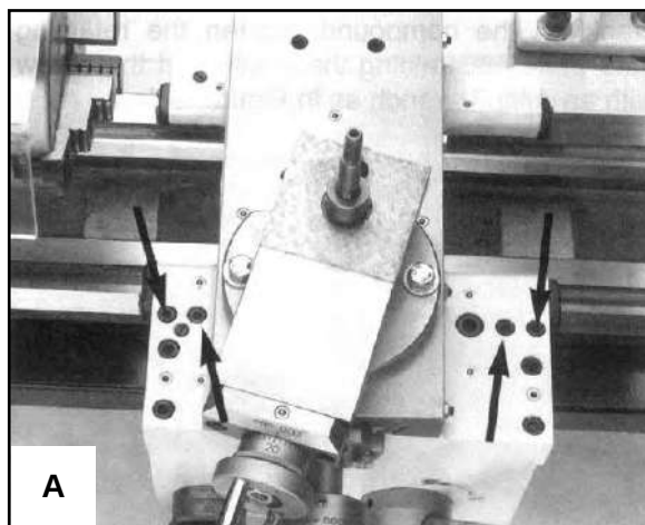
Figura 35 – Viti carrello (A: parte anteriore – B: parte posteriore).
