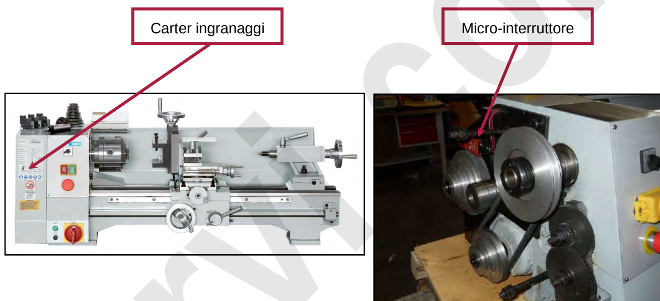
Figura 12 – Carter di protezione ingranaggi e cinghie.
