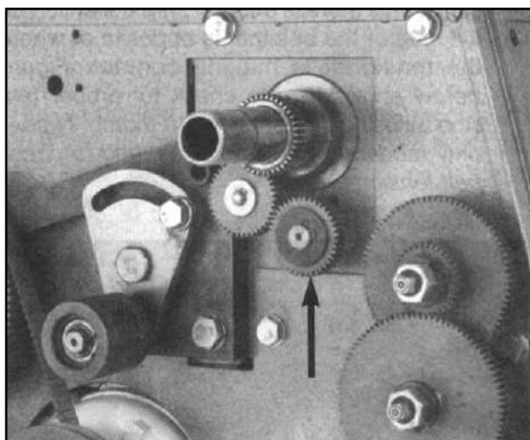
Figura 30 – Spostamento albero con ingranaggio.
