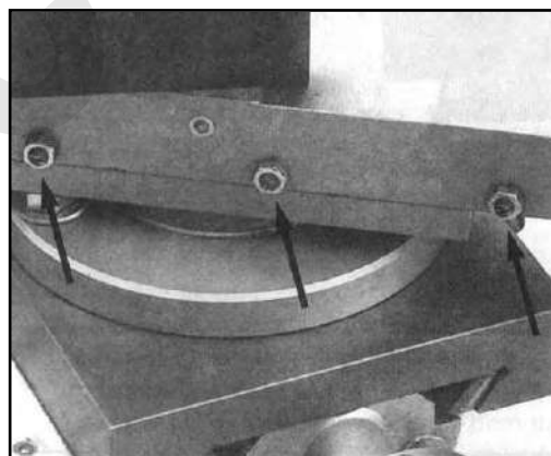
Figura 34 – Viti slitta longitudinale.
