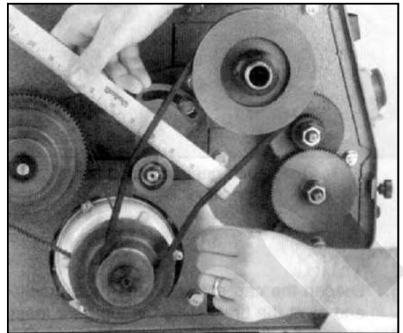
Figura 25 – Verifica tensione cinghia.
