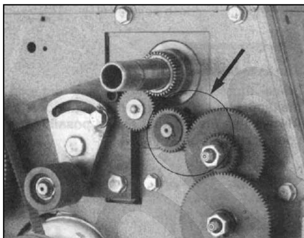
Figura 30 – Spostamento albero con ingranaggio.
