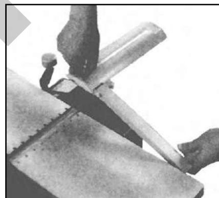
Figura 23 – Carter in posizione corretta per la configurazione “a spessore”.
