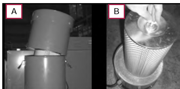
Figura 26 – Smontaggio del filtro ciclone
