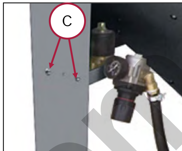
Figura 5 – Fissaggio gruppo pneumatico.
