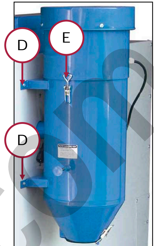
Figura 8 – Montaggio aspiratore.
