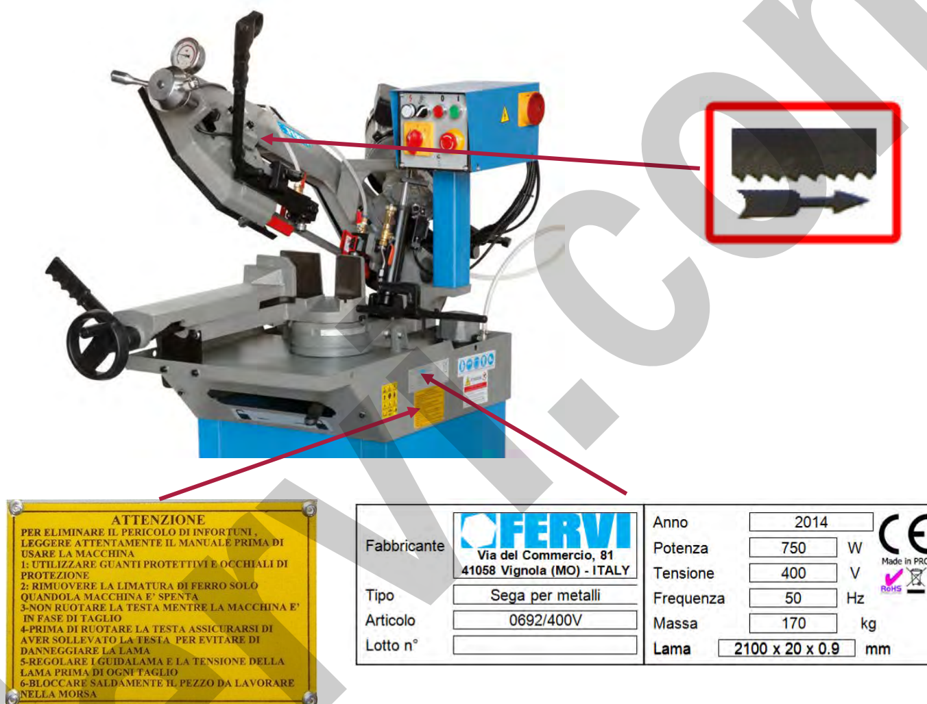
Figura 2 – Targhetta di identificazione e pittogrammi.
