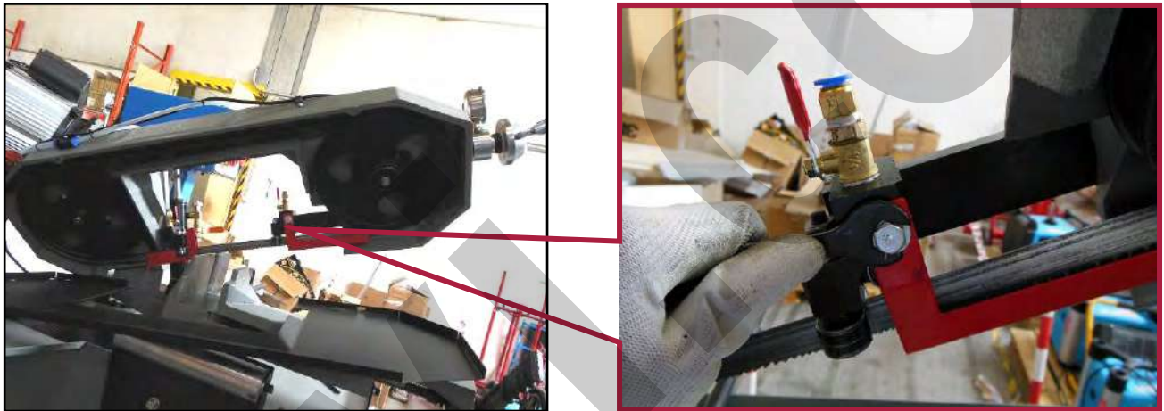
Figura 39 – Rimozione del guida lama.
