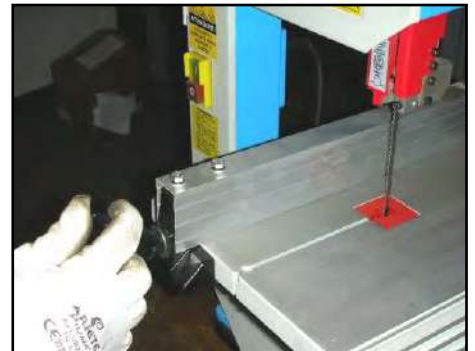
Figura 12 – Regolazione squadra.
