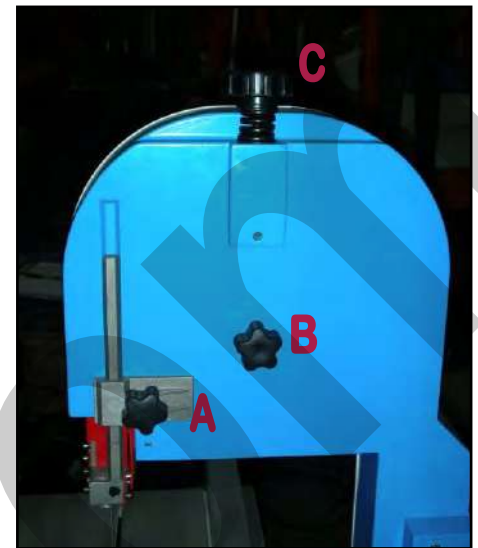
Figura 7 – Pomelli lato motore.
