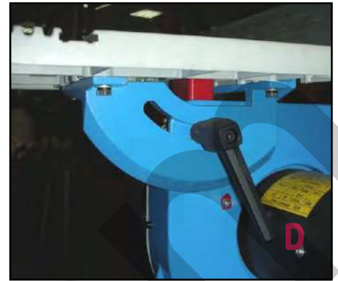
Figura 9 – Leva inclinazione tavola.
