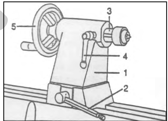
Figura 19 – Contro punta.
