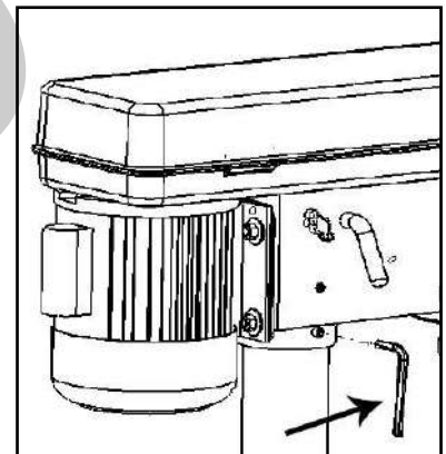
Figura 5 – Installazione testa
