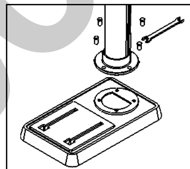
Figura 2 - Assemblaggio base
