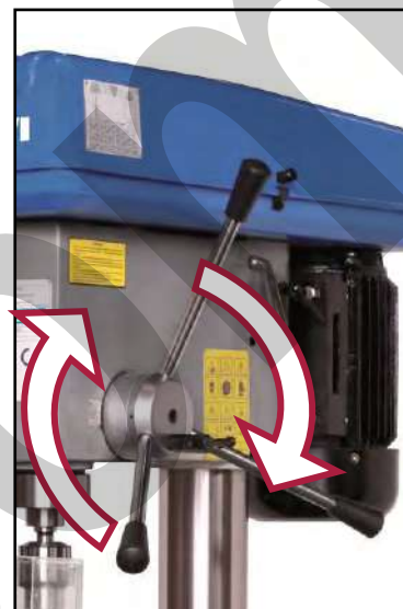
Figura 41 – Abbassamento mandrino
