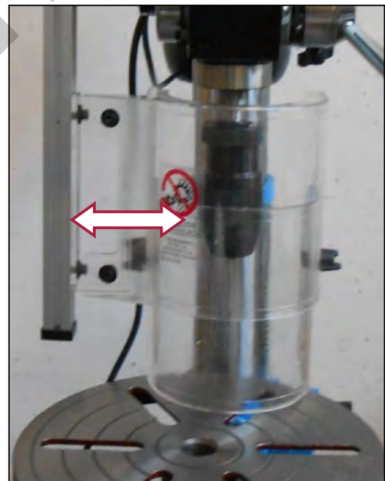
Figura 18 - Scorrimenti del riparo in senso verticale e longitudinale
