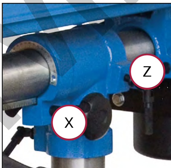
Figura 17 – Pomelli di regolazione della profondità.
