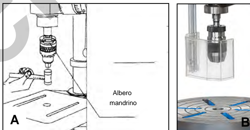
Figura 2 - mandrino (A: battere col martello – B: vista d'insieme).
