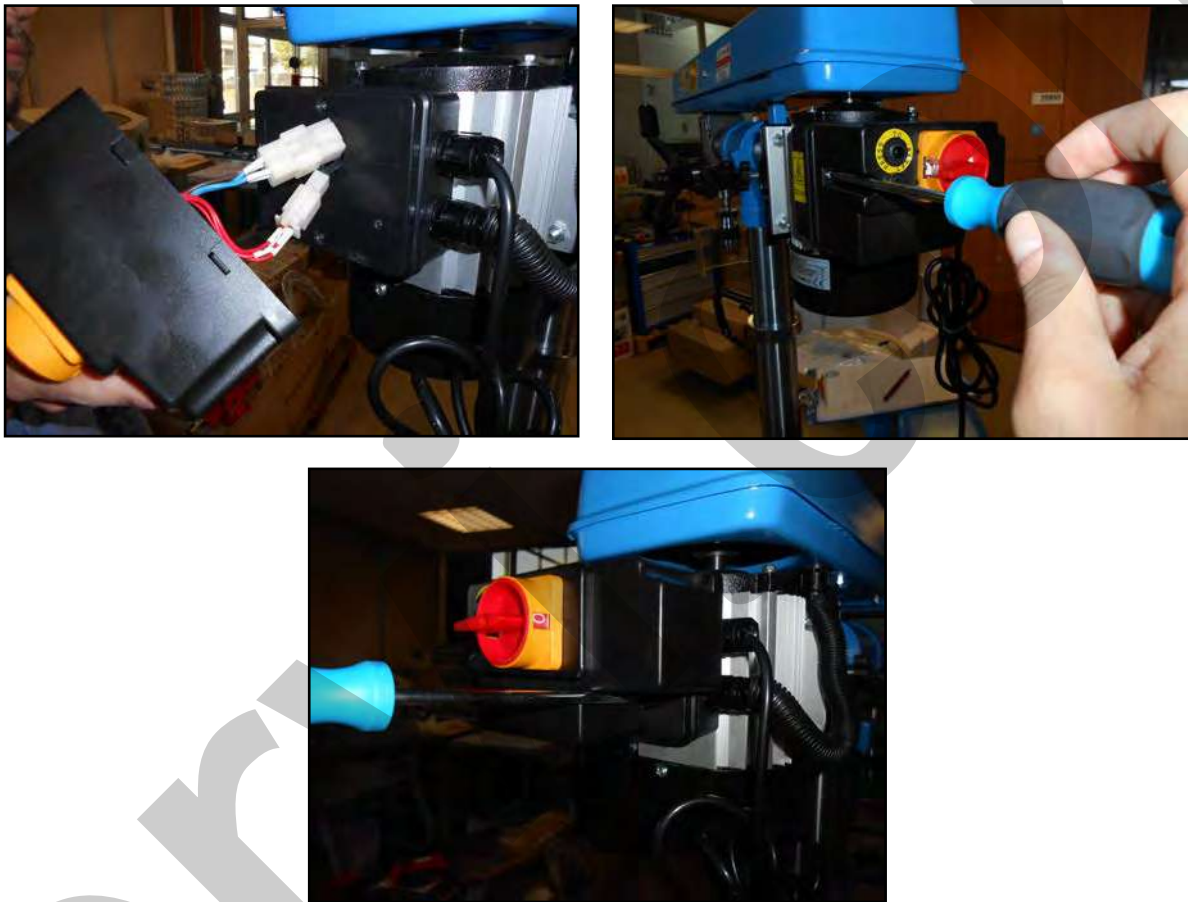
Figura 10 – Montaggio della scatola elettrica.
