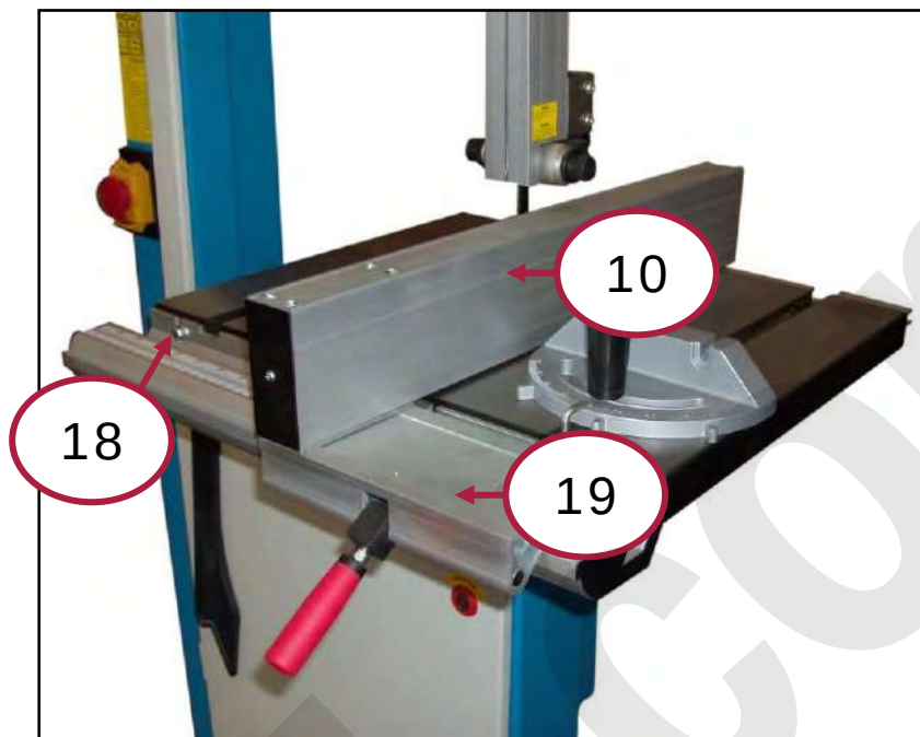
Figura 20 - Montaggio della squadra guida-pezzo.
