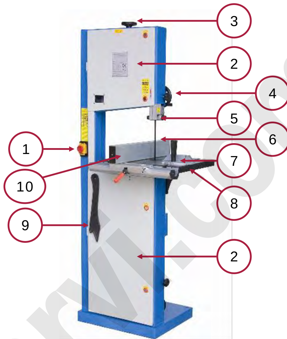
Figura 2 - Dettaglio delle parti principali.
