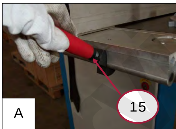
Figura 14 – Leva di fissaggio della squadra (A: Sbloccata – B: Bloccata).
