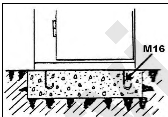
Figura 21 - Fori di fissaggio.
