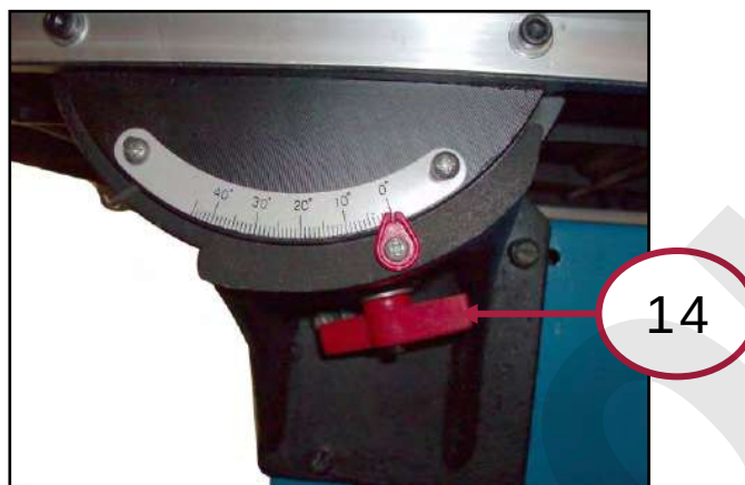
Figura 13 – Dado di bloccaggio inclinazione tavola.
