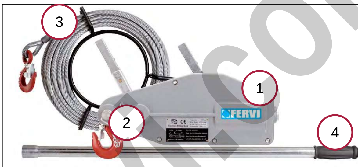
Figura 1 – Parti principali dell'argano.
