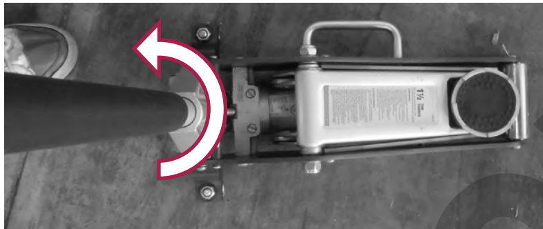
Figura 12 - Apertura valvola di ritegno.
