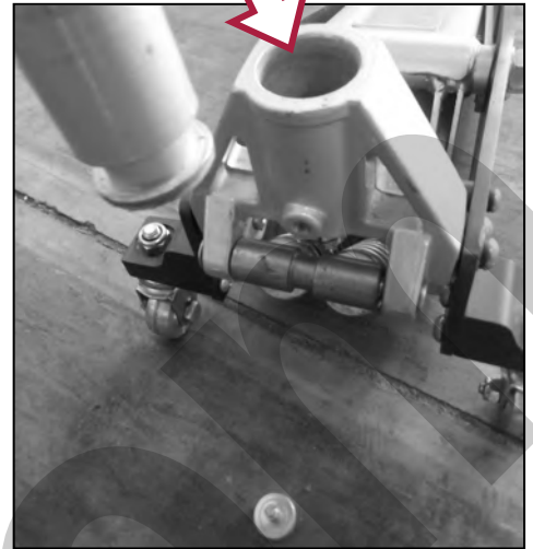
Figura 7 – Inserimento leva.
