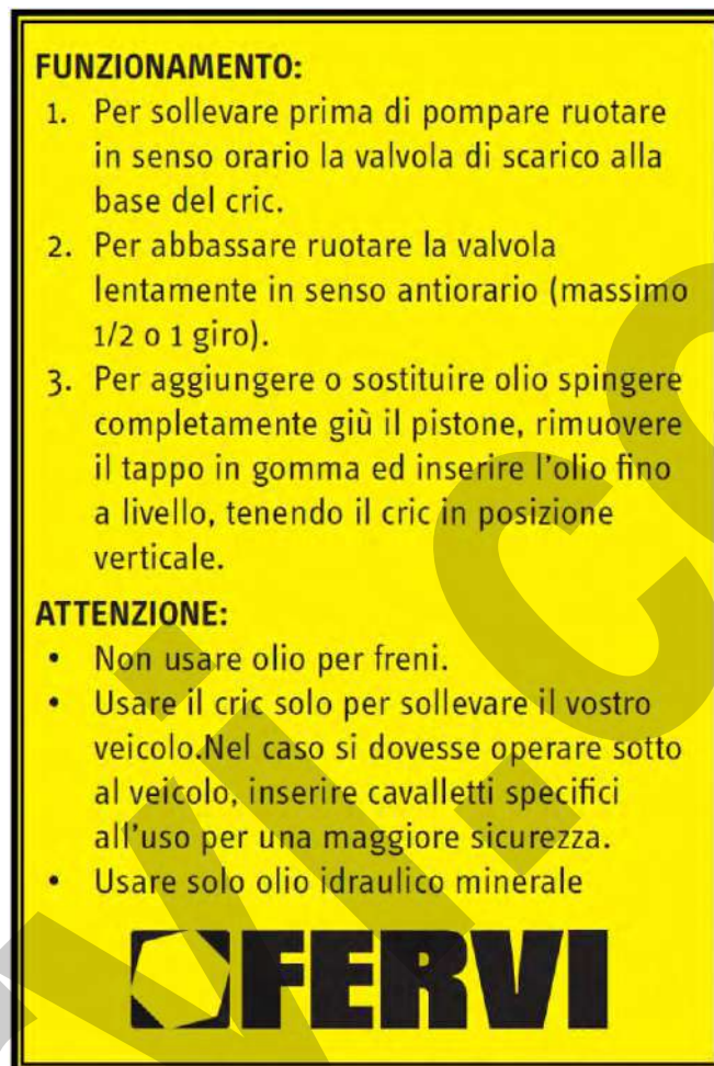
Figura 5 – Dettaglio pittogramma sul telaio del Cric a carrello.
