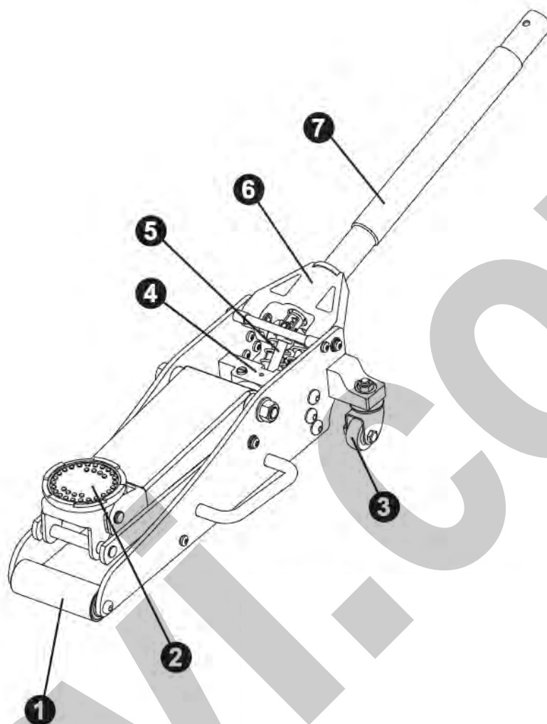
Figura 14 - Disegno esploso delle parti di ricambio del telaio.
