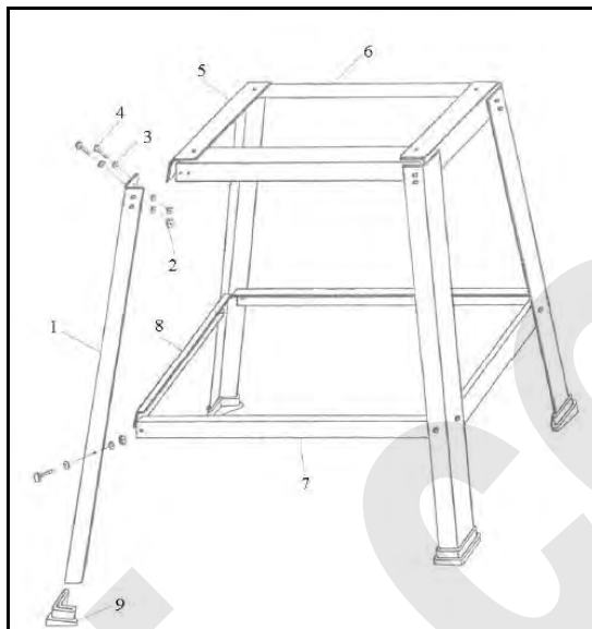
Figura 15 - Montaggio basamento.
