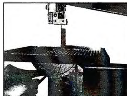
Figura 18 – Azzeramento tavola.
