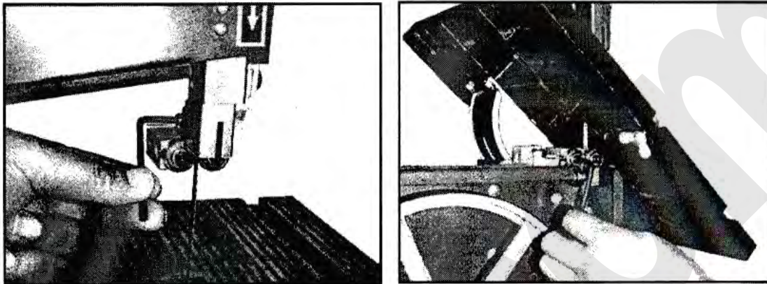
Figura 19 – Guida lama.
