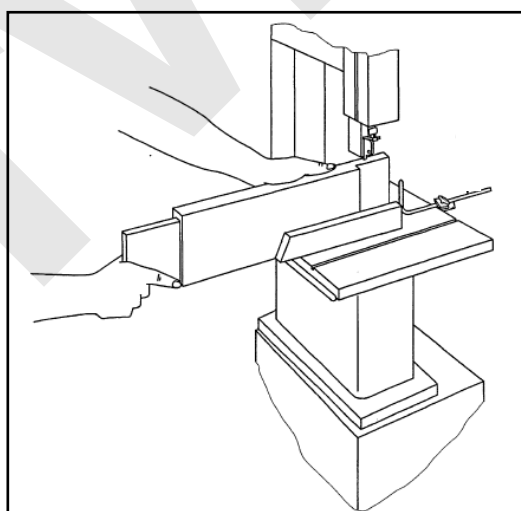
Figura 30 – Esecuzione di scanalature.
