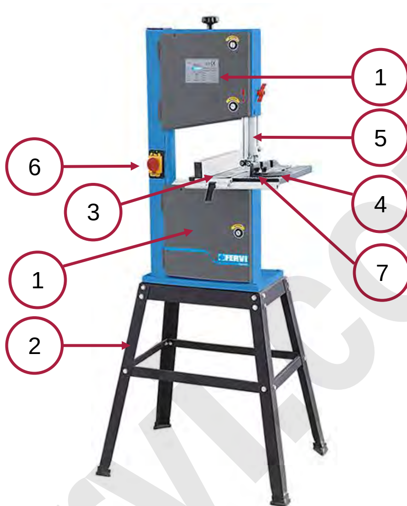
Figura 1 - Dettaglio delle parti principali.
