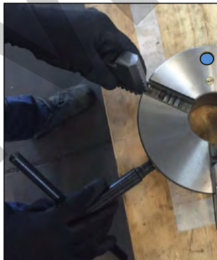
Figura 7 – Inserimento delle altre griffe
