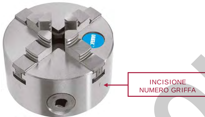
Figura 6 – Incisione del numero griffa
