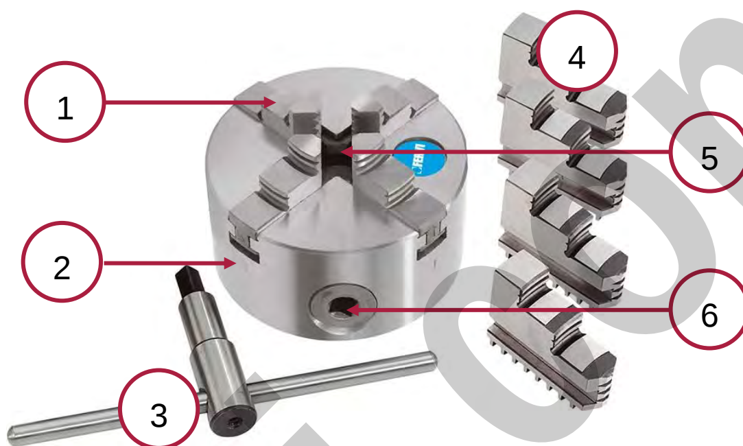
Figura 2 – Parti del mandrino
