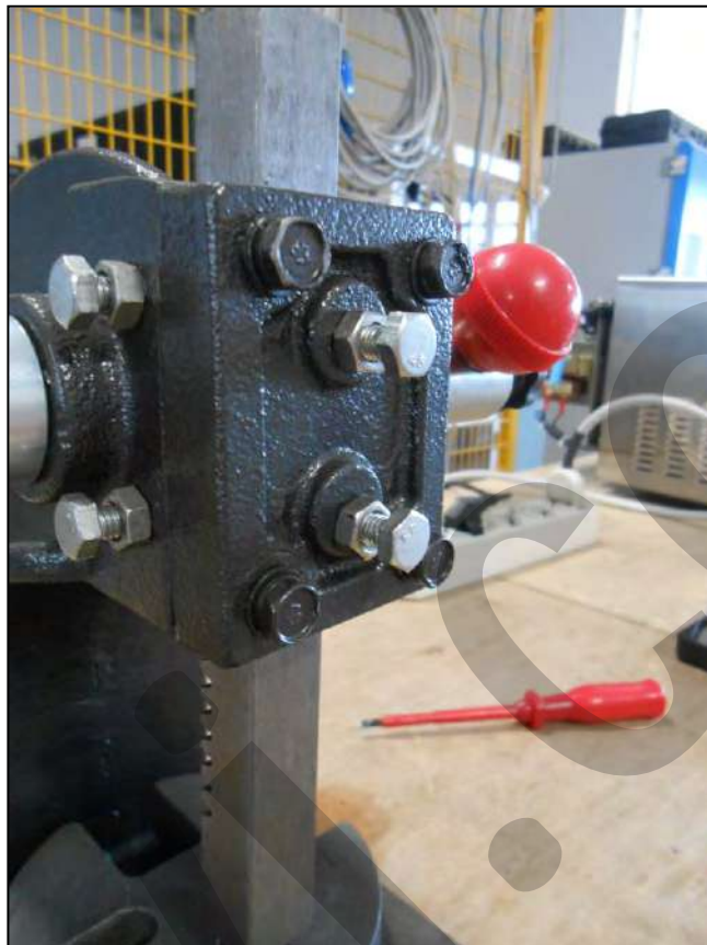
Figura 6 – Regolazione guide scorrimento.
