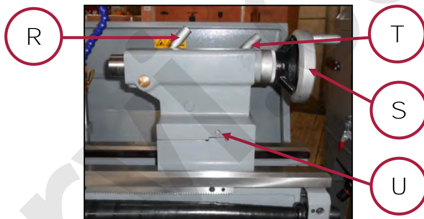
Figura 26 - Leva e volantino della contropunta.
