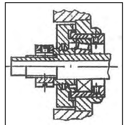
Figura 36 – Allineamento mandrino.
