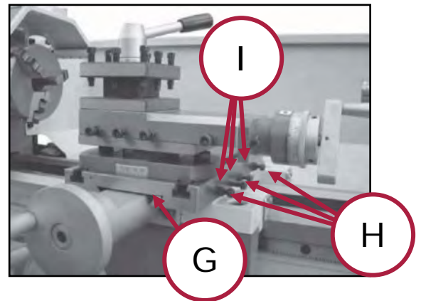
Figura 39 – Slitta trasversale.
