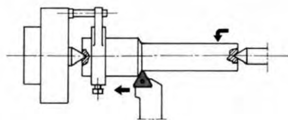
Figura 35 – Tornitura tra centri.
