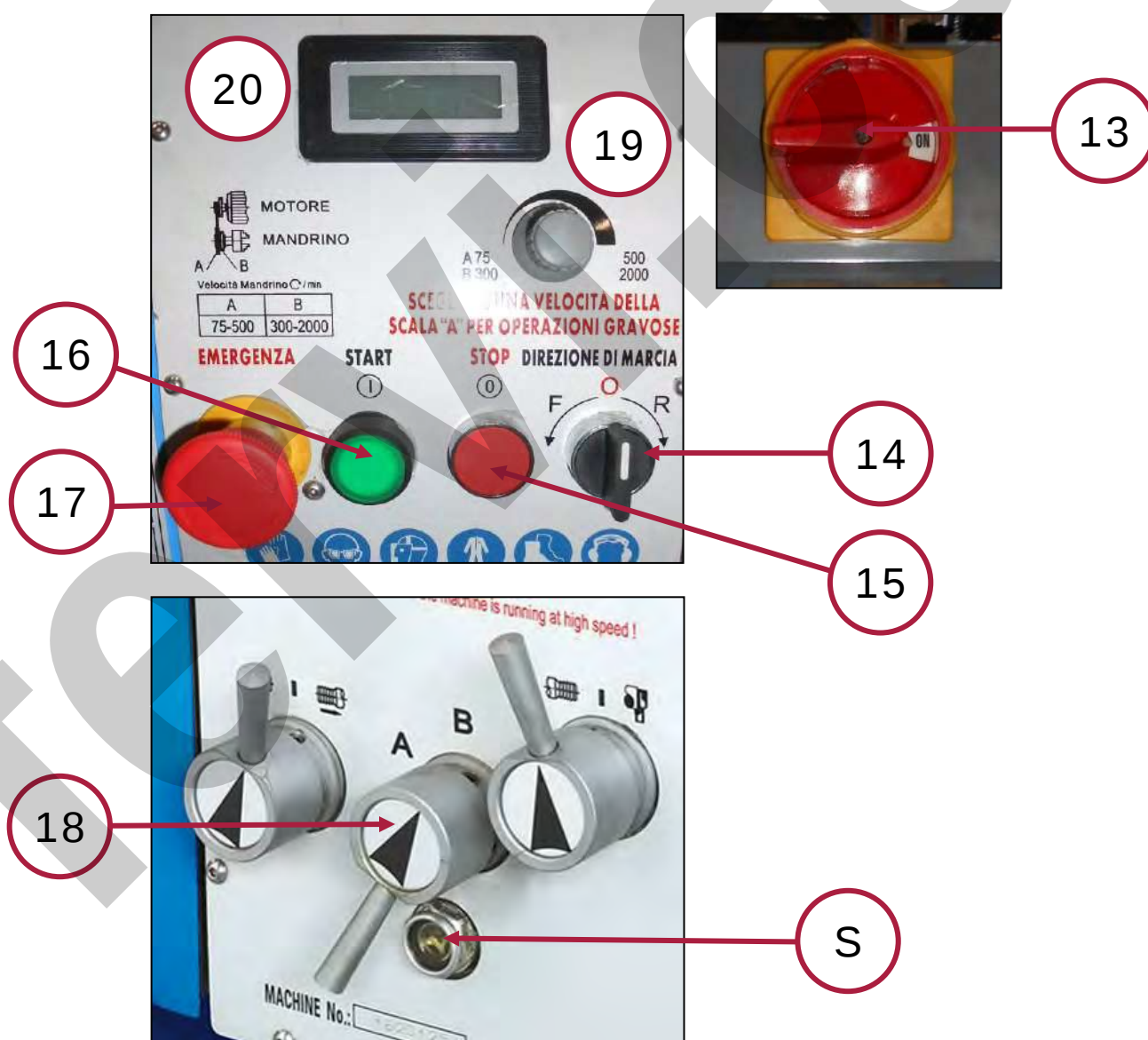
Figura 14 - Quadro di comando.
